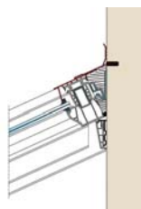
Dachanschluss
