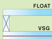
Verbund – Sicherheitsglas als Durchbruch- und Absturz-sicherung
