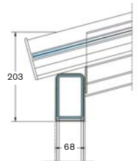
Traufpunkt ohne Regenrinne
