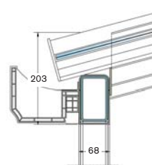
Traufpunkt mit Regenrinne
